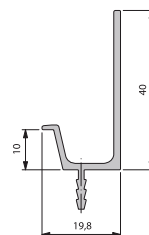
ידית סירה 40 (H-18) גימור טבעי או ברק משי
