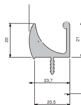
ידית חבצלת 20 (H-1) גימור טבעי
